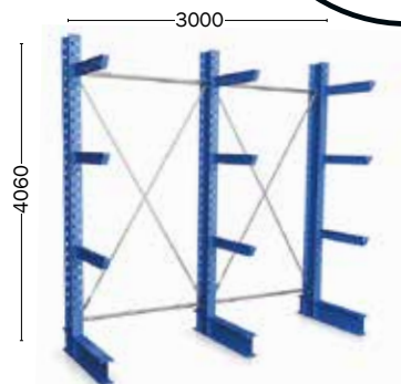
Esimerkki 1 1-puoleinen, 3-pylvästä Jalka + 3 uloketasoa Korkeus 4060 mm (pylväs IPE220)
